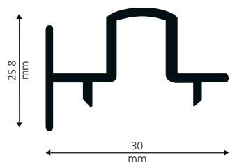
Adaptador EMF8165
